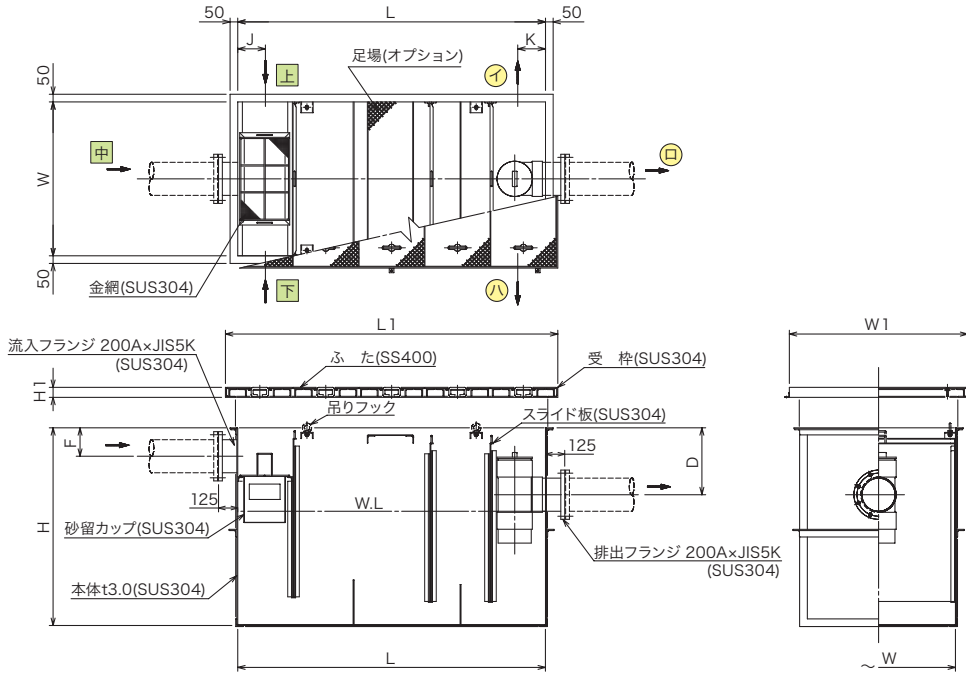
構造図
