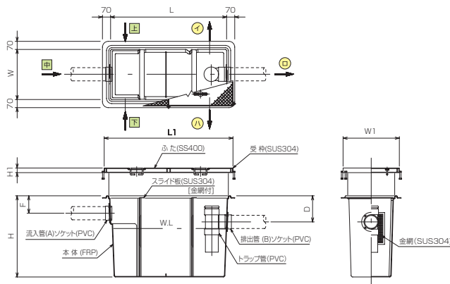
構造図
