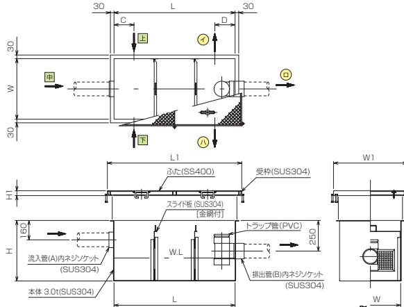
構造図
