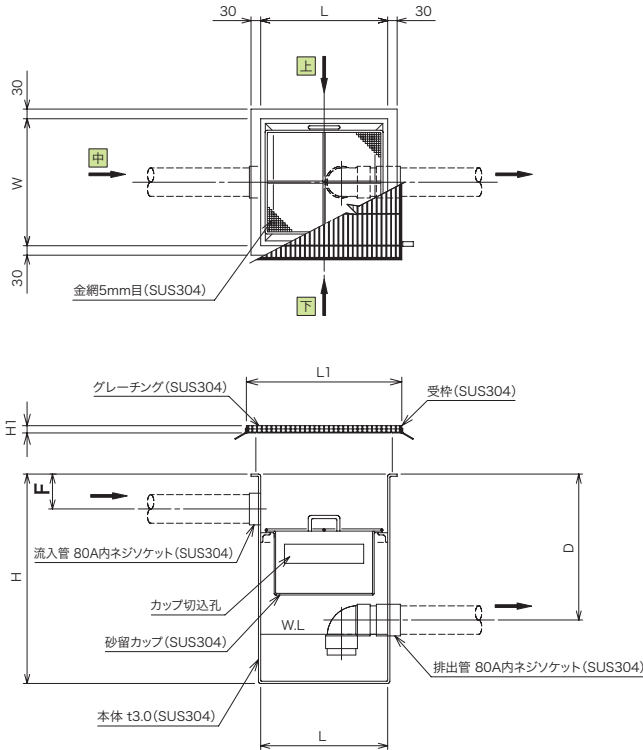
構造図
