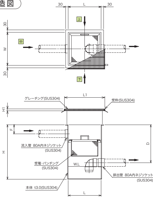
構造図
