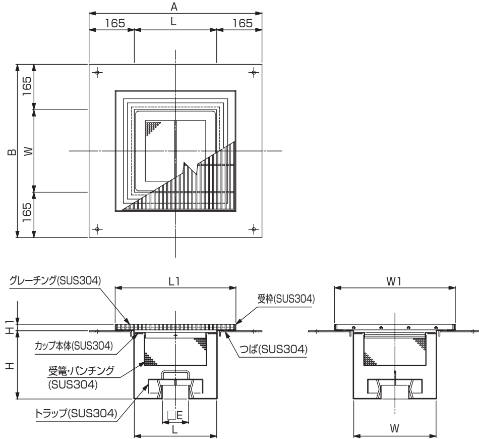
構造図
