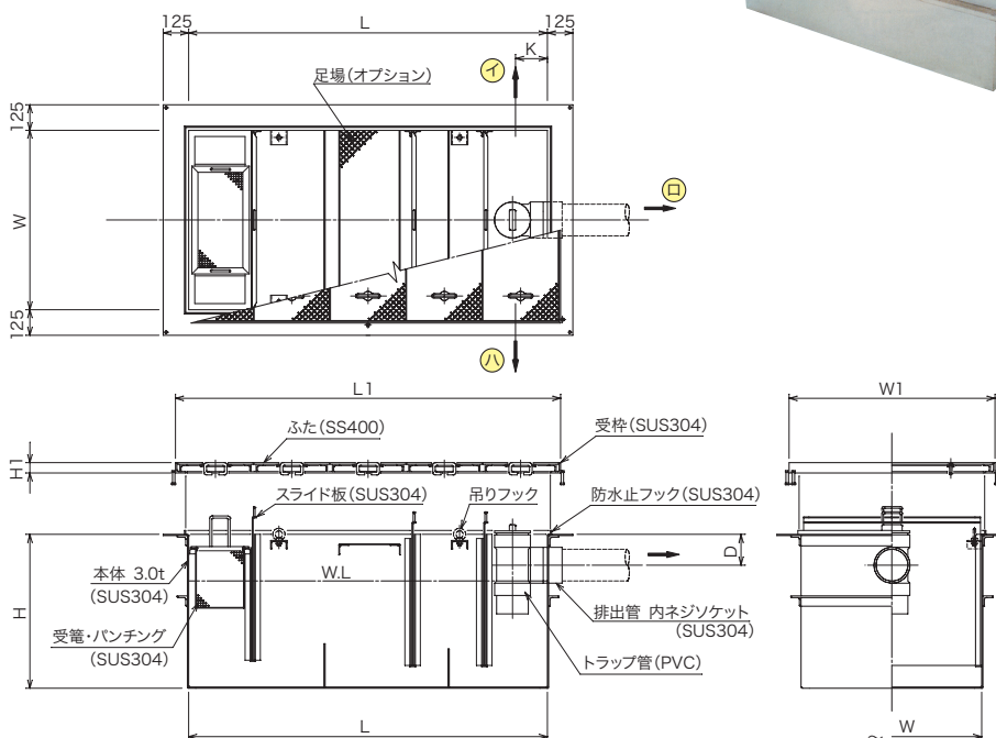
構造図
